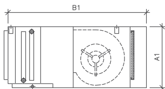
EMBOCADURA ASPIRACION Y ACCESO LATERAL O INFERIOR FILTRO
