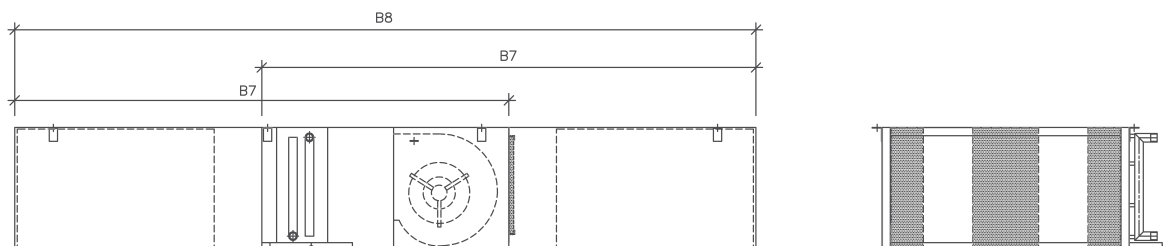
PLENUM DE SILENCIADOR EN IMPULSION Y/O ASPIRACION
